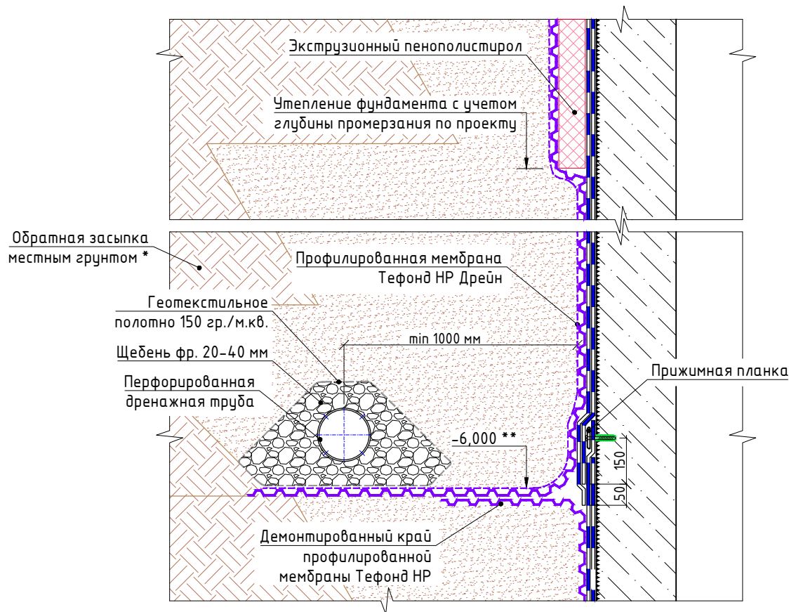
2 Этап. Устройство промежуточного дренажа
